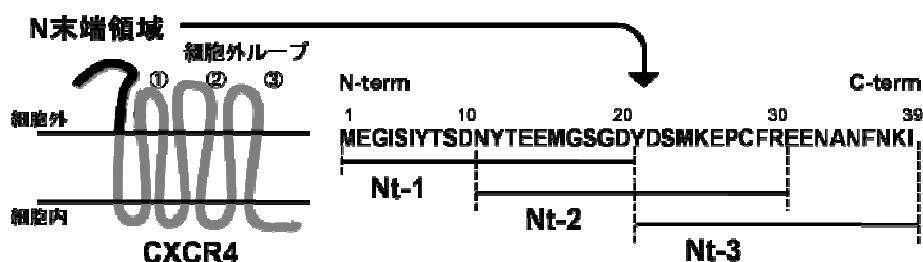
図. 3 種類の CXCR4 N 末端領域断片ペプチド
